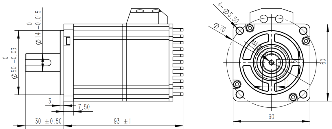
图 1-4 UM6020C-2ED1A 安装尺寸图 (mm)
