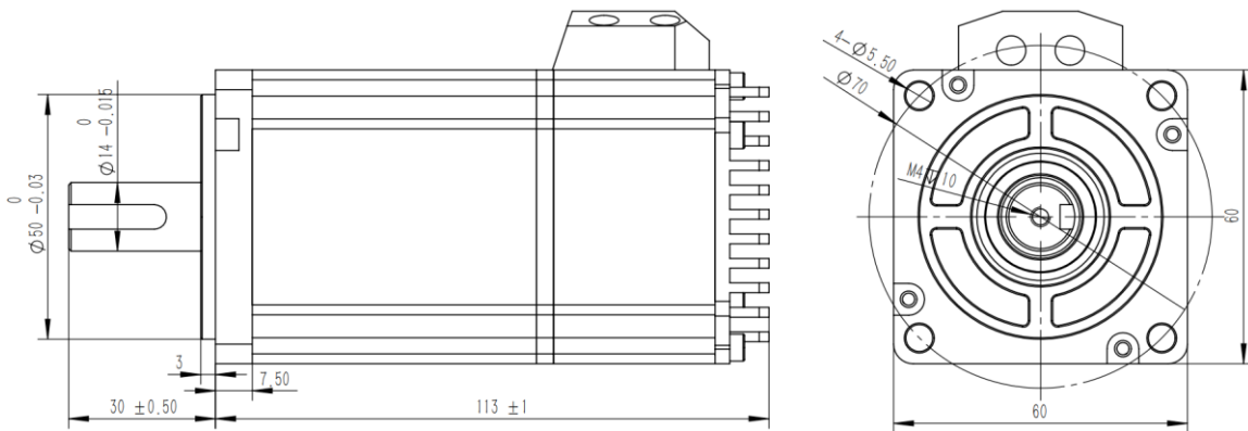
图 1-5 UM6020C-2ED1A-G 安装尺寸图 (mm)
