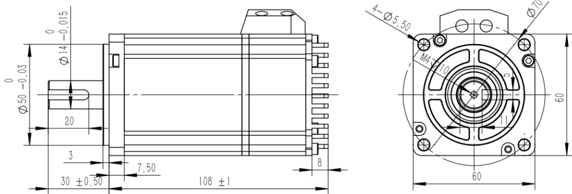
图 1-6 UM6040C-2BB0A 安装尺寸图 (mm)
