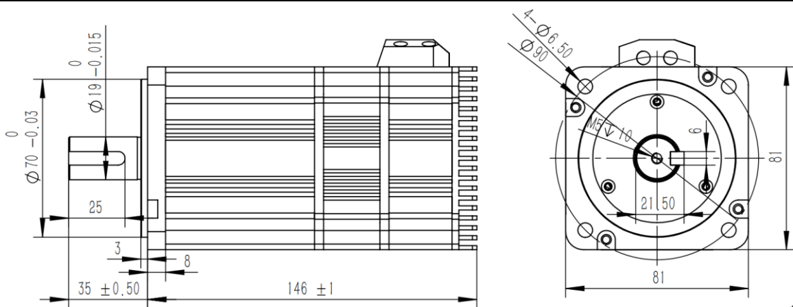
图 1-12 UM8075C-2BB0A-G 安装尺寸图 (mm)
