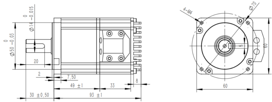
图 1-4 UM6020C-2DD1A 安装尺寸图 (mm)
