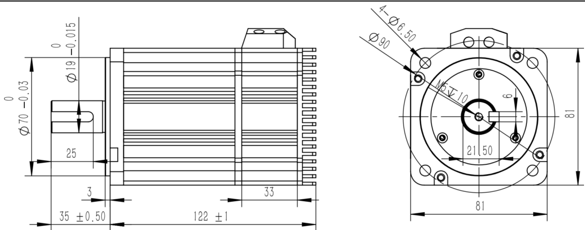
图 1-11 UM8075C-2ED1A 安装尺寸图 (mm)
