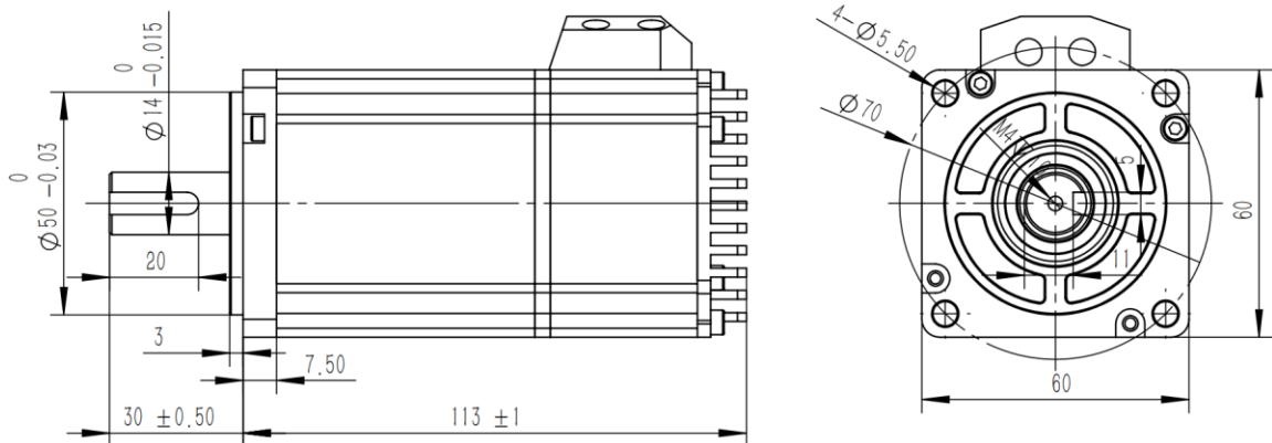
图 1-9 UM6040C-2ED1A 安装尺寸图 (mm)
