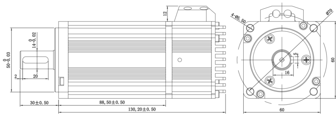
图 1-3 UM6040C-2AA0A 安装尺寸图 (mm)
