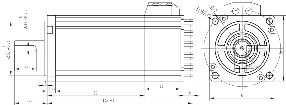
图 1-10 UM6040C-2ED1A-G 安装尺寸图 (mm)
