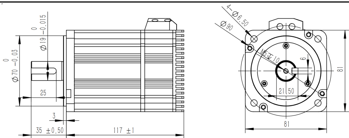
图 1-11 UM8075C-2BB0A 安装尺寸图 (mm)
