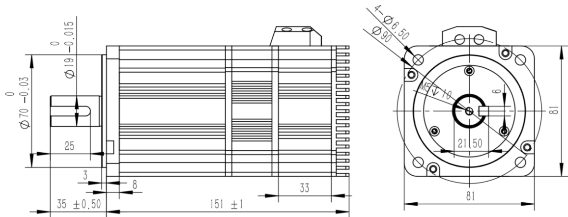
图 1-12 UM8075C-2ED1A-G 安装尺寸图 (mm)
