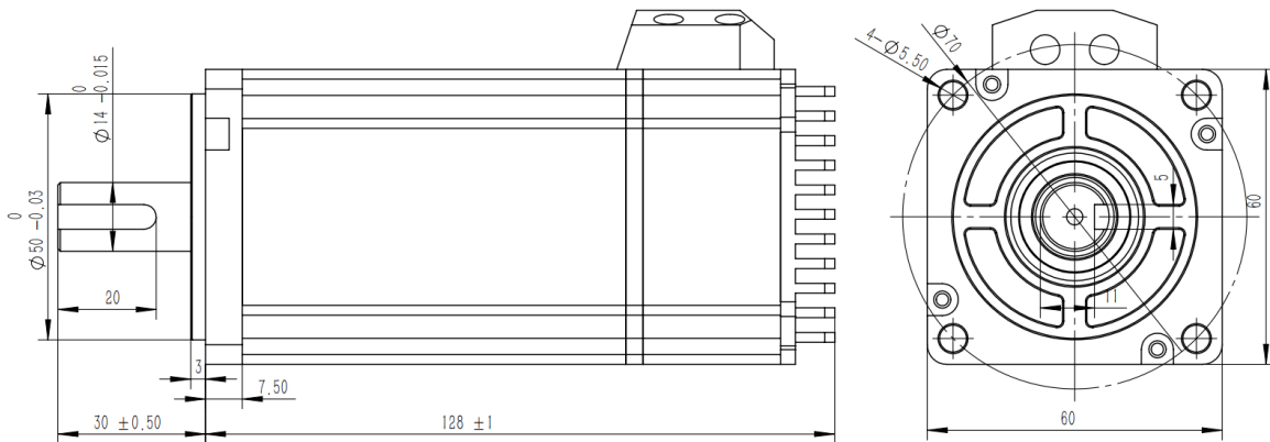
图 1-7 UM6040C-2BB0A-G 安装尺寸图 (mm)
