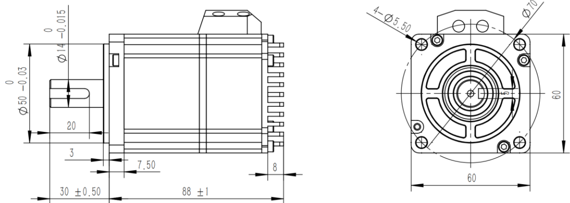
图 1-4 UM6020C-2BB0A 安装尺寸图（mm）
