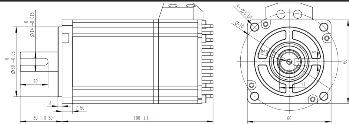
图 1-5 UM6020C-2BB0A-G 安装尺寸图（mm）
