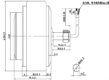
□ UM10540NB0A2533F30--S机械尺寸图 (单位: mm)
