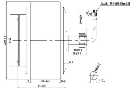
□ UM10550NB0A3027C30-S机械尺寸图 (单位: mm)
