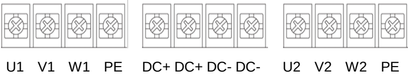
图 2-1 RS20270H 主回路端子
