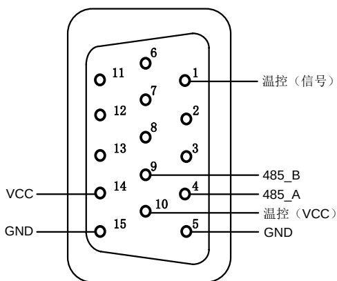
DS20270H 编码器接口的管脚定义
