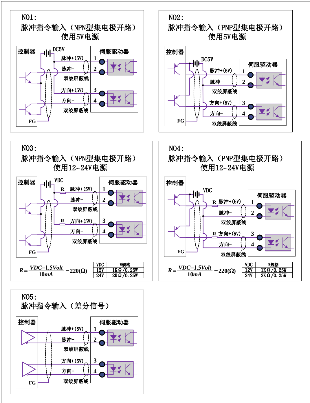
图 2-7 脉冲指令输入接线图
