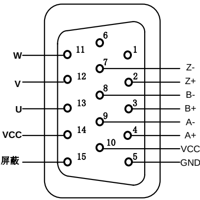
图 2-3 RS20270H 编码器的管脚定义
