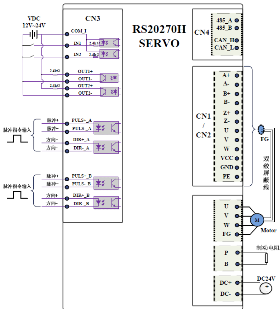
图 2-6 驱动器外部接线图
