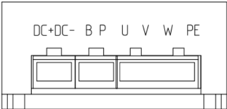
图 2-1 DS/RS10240E
