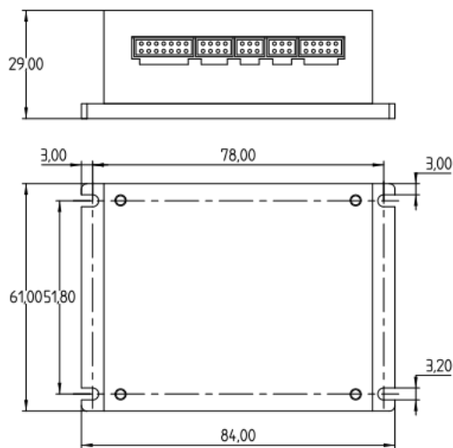
图 1-2 DS/RS10240E 安装尺寸图（mm）
