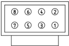
图 2-5 CN6 管脚（母座）
