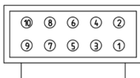
图 2-3 CN3 管脚（母座）
