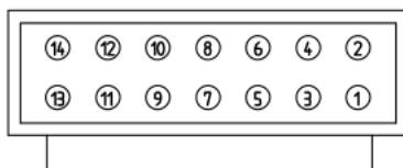
图 2-4 CN4 管脚（母座）
