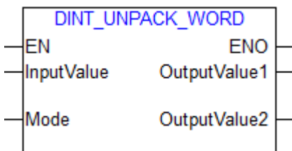
图 101 DINT_UNPACK_WORD 功能块
