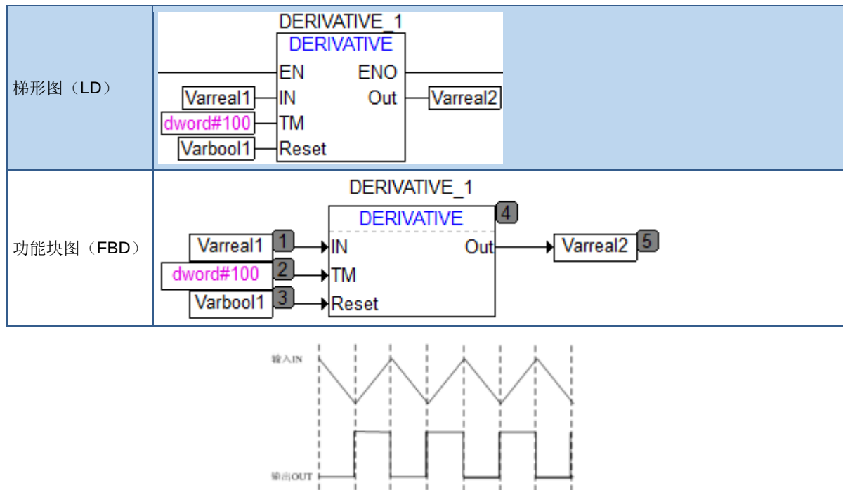
图 107 输入输出对应关系
