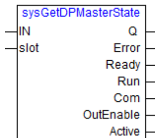
图 143 sysGetDPMasterState 指令
