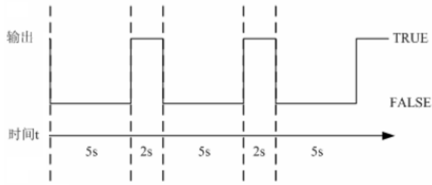
图 116 输出波形
