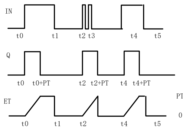
图 92 TP 的时序图
