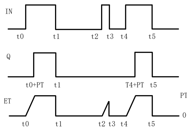
图 87 TON 的时序图
