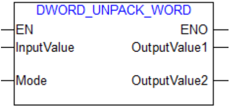
图 100 DWORD_UNPACK_WORD 功能块
