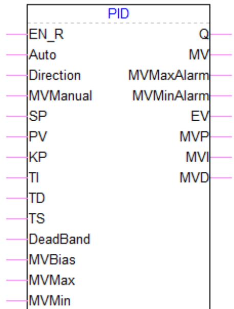
图 113 PID 功能块
