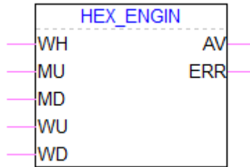
图 129 HEX_ENGIN 功能块
