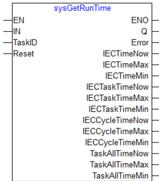
图 141 sysGetRunTime 指令
