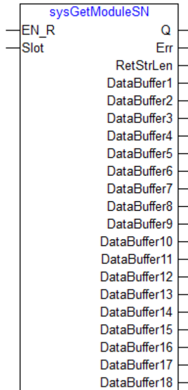
图 140 sysGetModuleSN 指令
