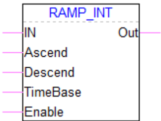
图 121 RAMP_INT 功能块
