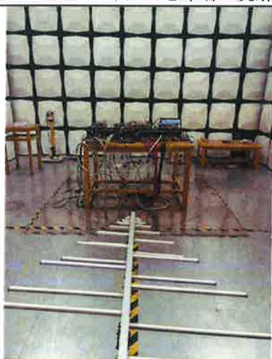
图11机箱端口发射 (30MHz ~ 1GHz)
