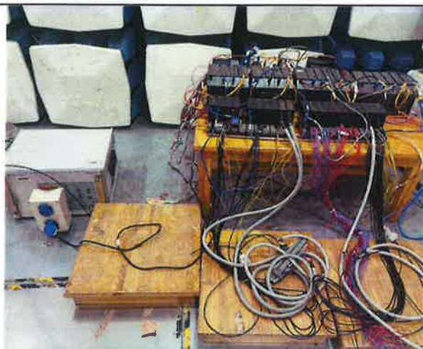
图9 电源端口发射
