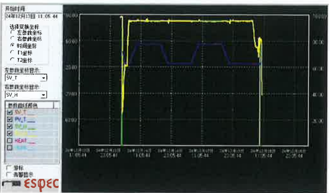
样品温度变化试验的曲线
