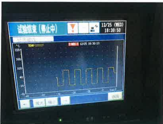
样品温度冲击试验的曲线 (1)
