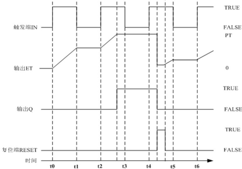
图 5-11-1 HS_TONR 时序图
