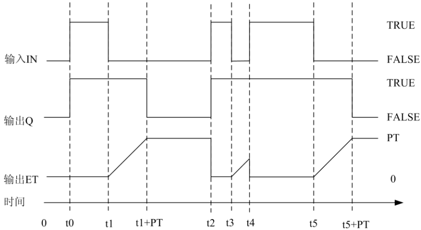
图 4-25-3 TOF 时序图
