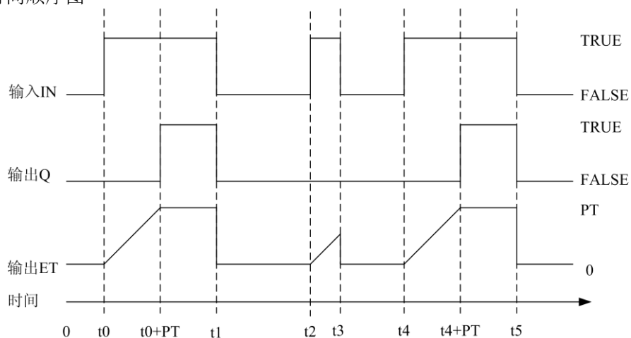
图 4-25-2 TON 时序图
