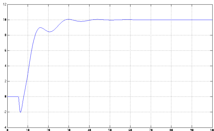
图 4-18-1 PD 调整的波形
