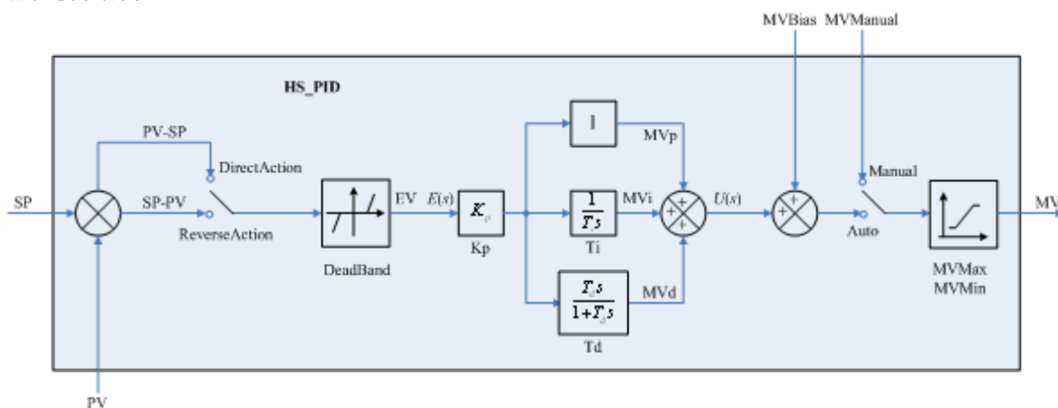
图 5.9.1-1PID 逻辑结构图
