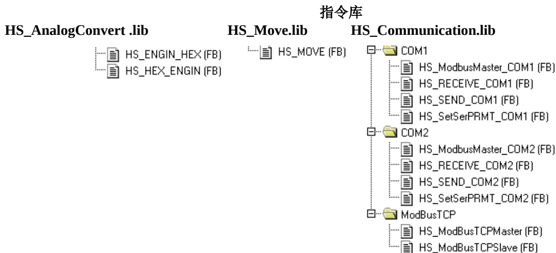
图 1-2-6 扩展指令
