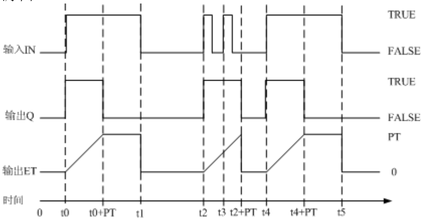
图 4-25-1 TP 时序图
