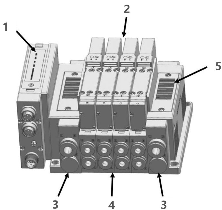
图 1.1.1 部件说明示意图
