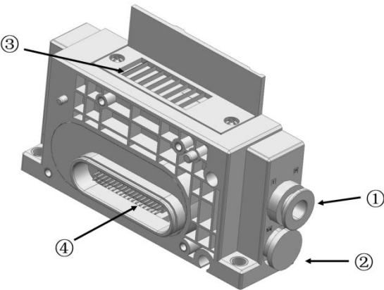
2.2.1 供气端板示意图
