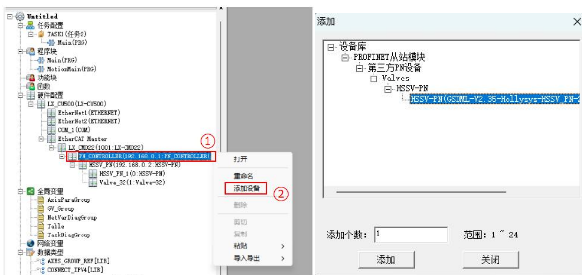
图 6.2.3 添加 PN 从站设备阀岛
