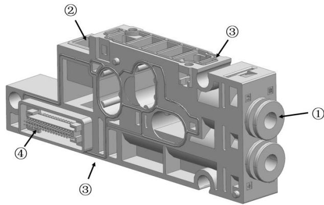
图 2.2.2 电磁阀底座
