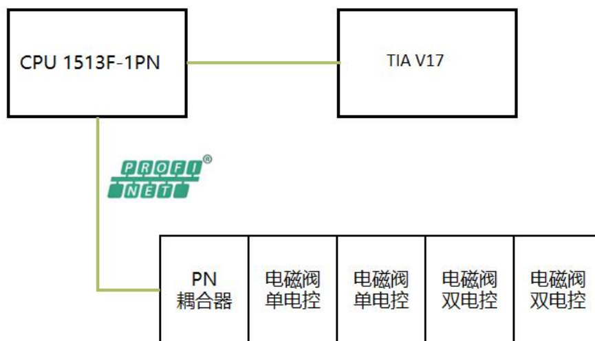
图 6.1.1 通信连接图
