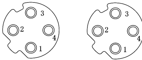
图 2.1.3 通信接口定义图
