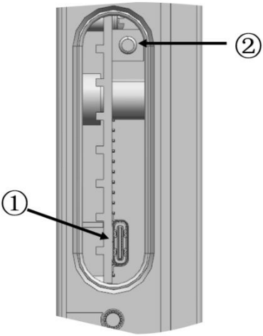
图 2.1.5 操作仓接口
