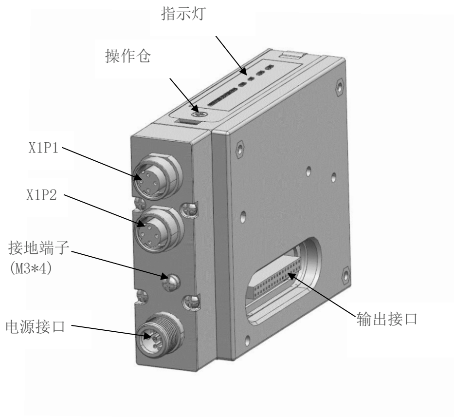
图 2.1.1 部件说明示意图
