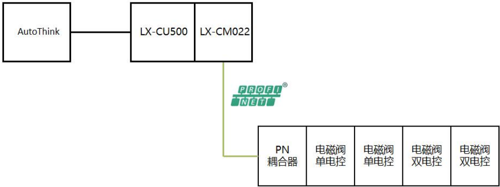
图 6.2.1 通信连接图
