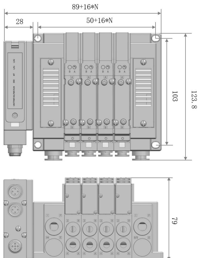
图 4.1.1 整体尺寸
