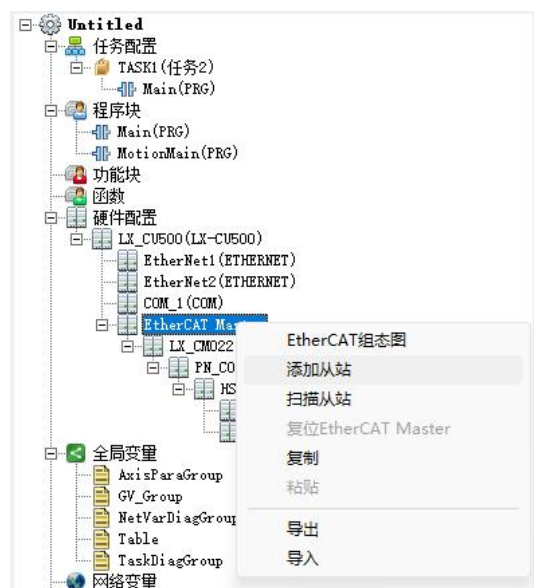
图 6.2.2 配置 LX-CM022 PN 主站模块
