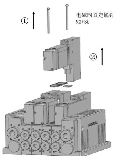
4-2-4 接头更换示意图
