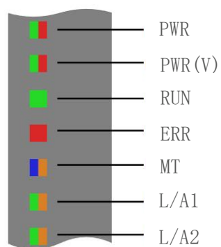
图 2.1.2 指示灯示意图
