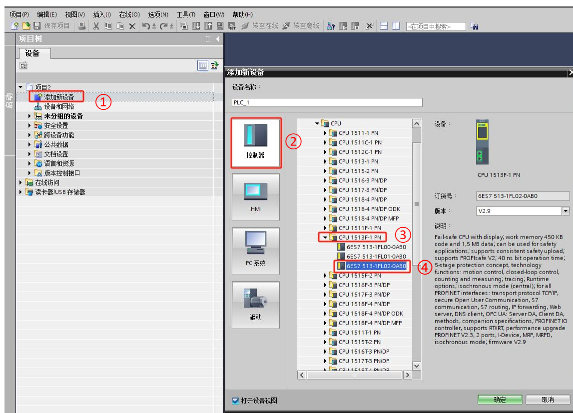
图 6.1.3 新建工程
