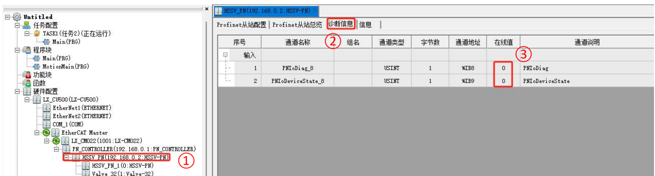
图 6.2.5 PN 从站诊断信息
