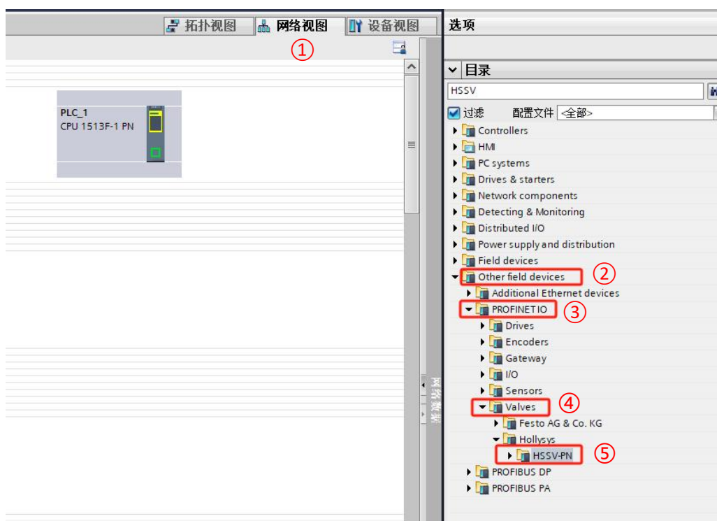
图 6.1.4 组态设备
