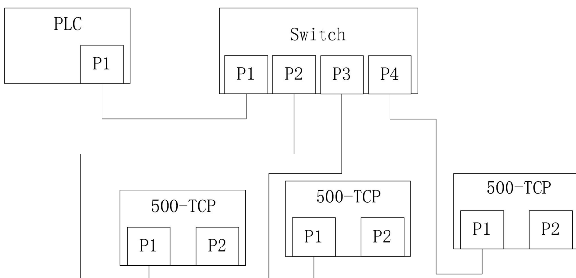
(b) 星型
