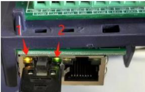
图 7-6 网口指示灯
