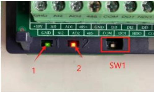
图 7-7 PN 卡指示灯及选择开关
