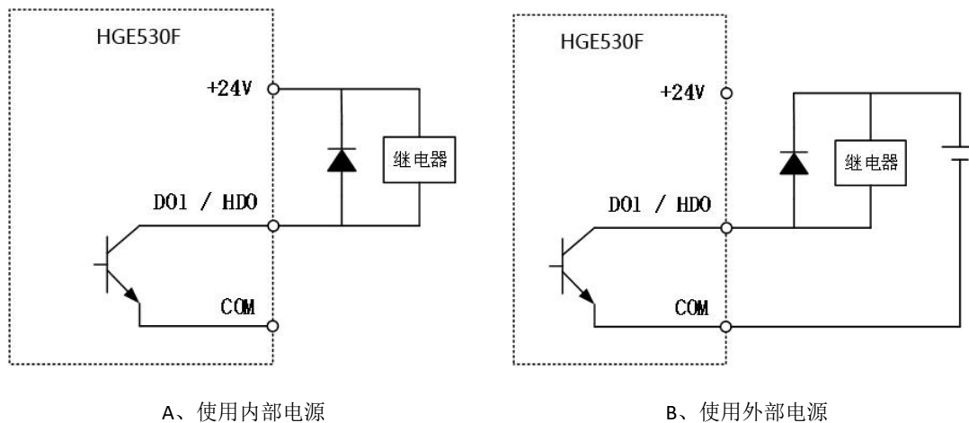
图 3-11 开关量输出端子接线图
