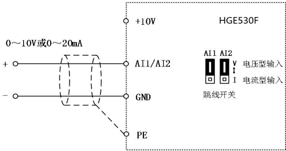
图 3-8 模拟量输入端子接线图
