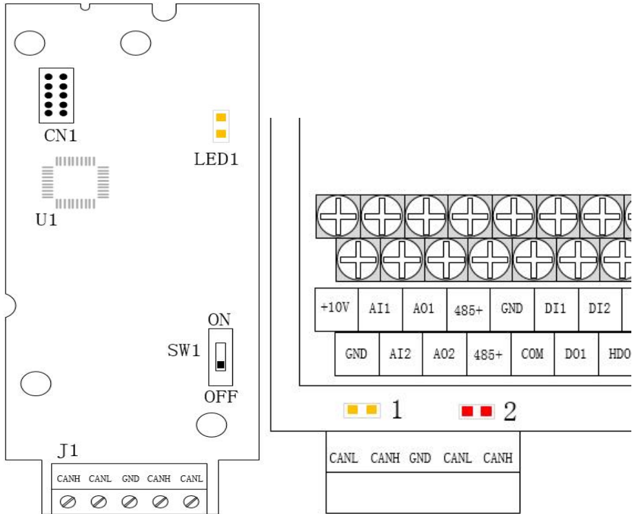
图 7-4 CANopen 通信卡及安装示意图
