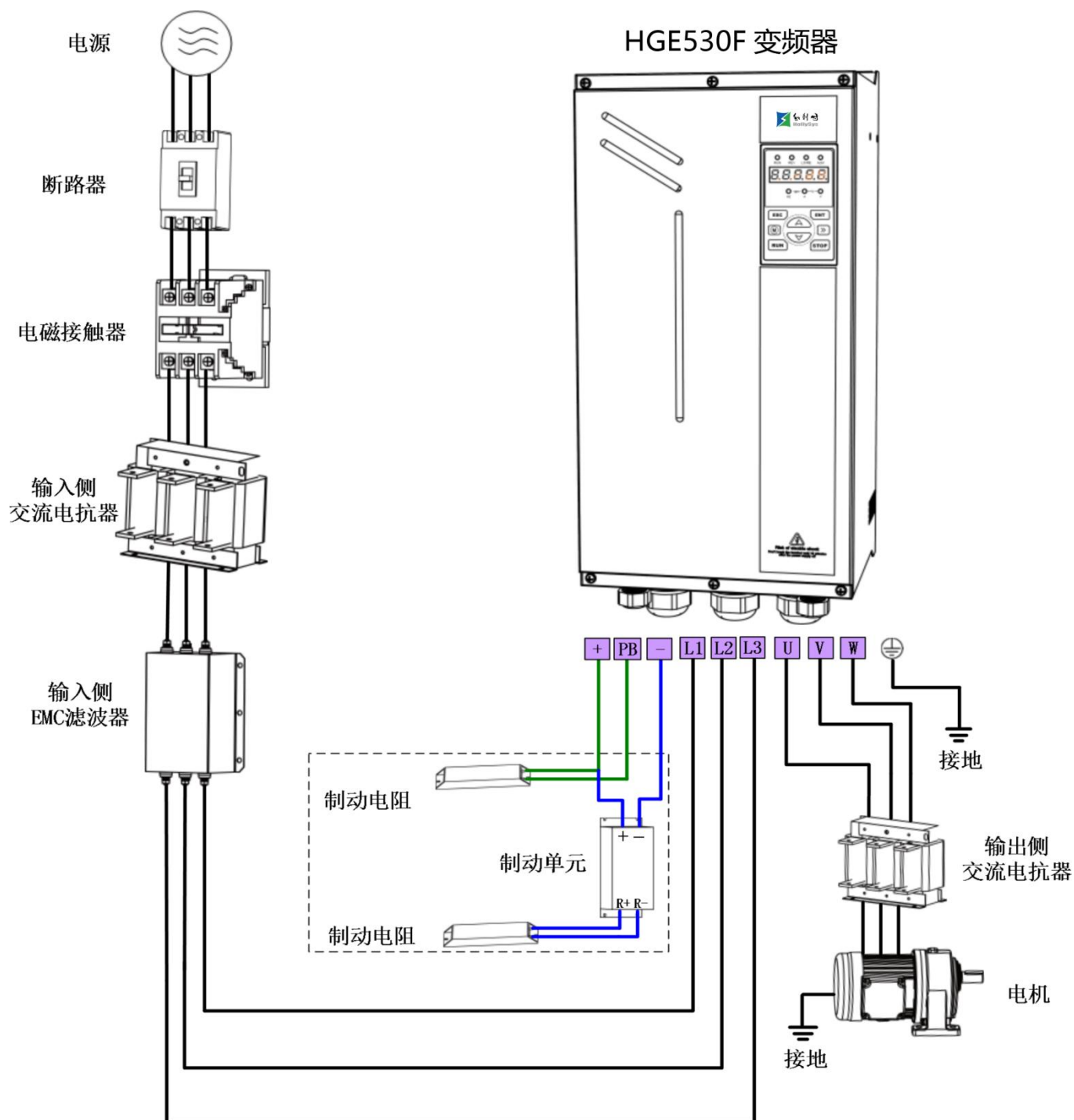
图 3-3 主回路接线图
