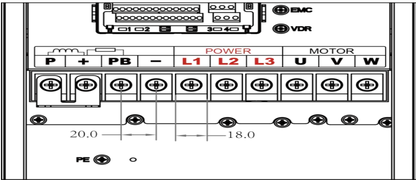
图 3-5 SIZE C~D 主回路接线端子示意图
