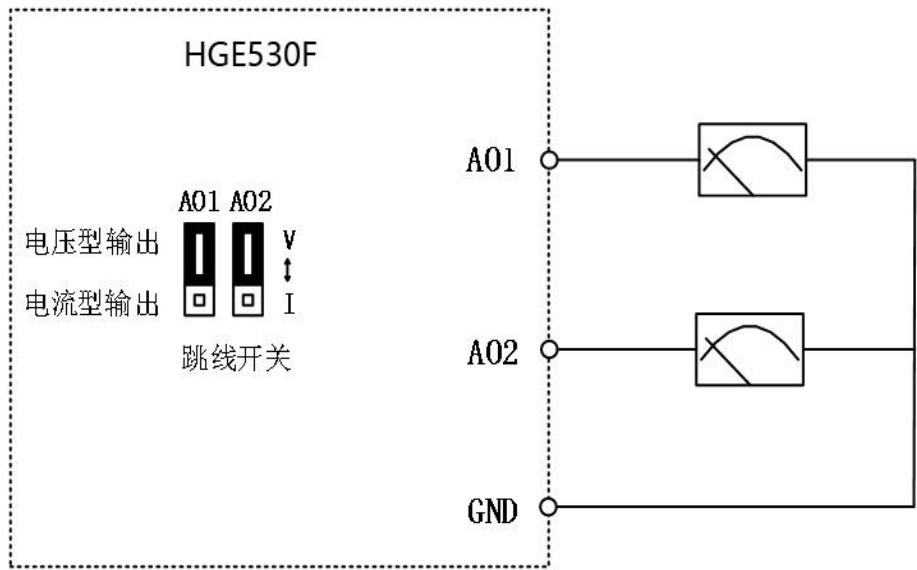
图 3-9 模拟量输出端子接线图
