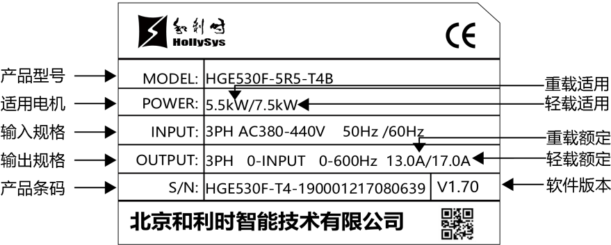
图 2-1 铭牌
