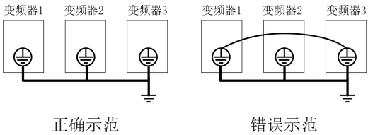
图 3-19 接地线接法示意图
