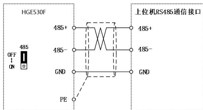
图 3-12 单台变频器 RS485 直接与上位机连接通信（不接终端电阻）
