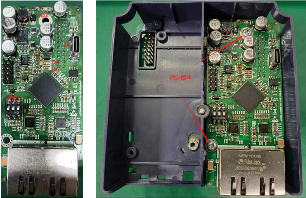
图 7-8 Modbus-TCP 通讯卡外观图与安装示意图
