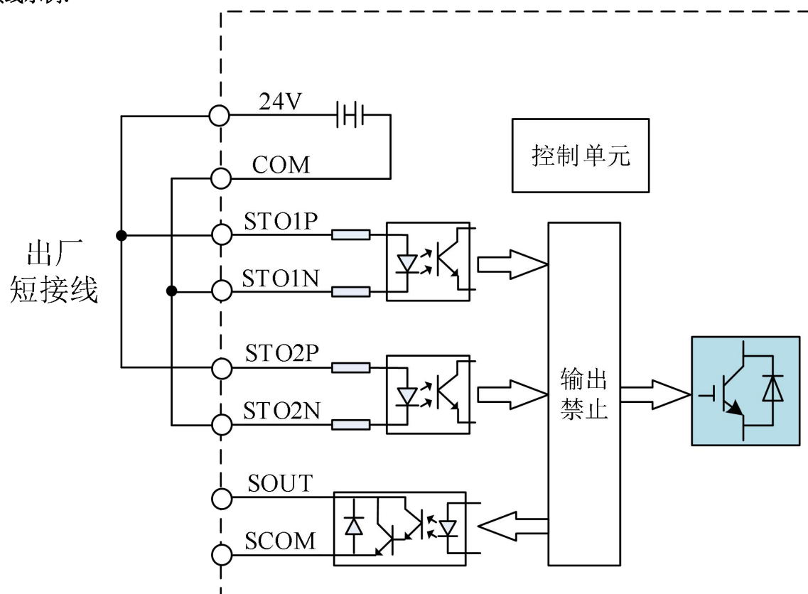
图 3-14 不使用 STO 功能接线图
