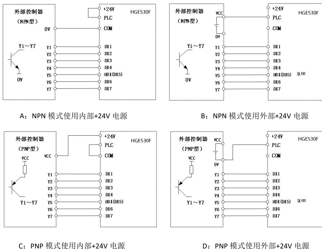
图 3-10 开关量输入端子接线图
