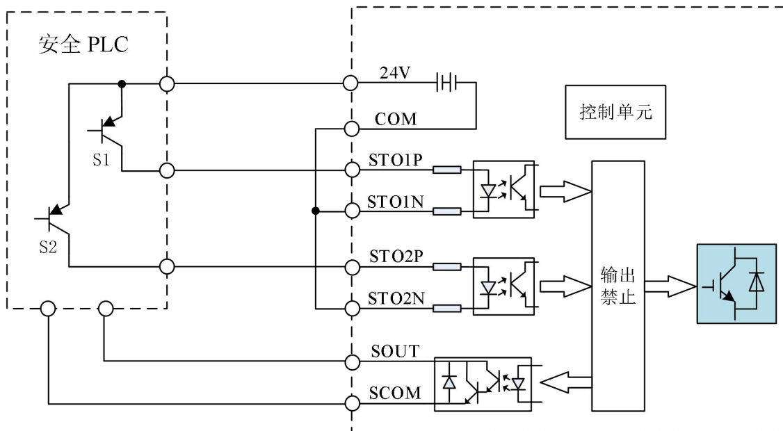
图 3-16 STO 与安全 PLC 接线图(内部 24V、PNP)
