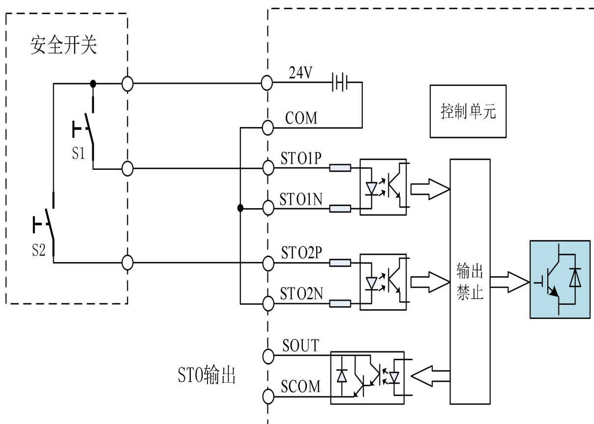
图 3-15 STO 与安全开关接线图
