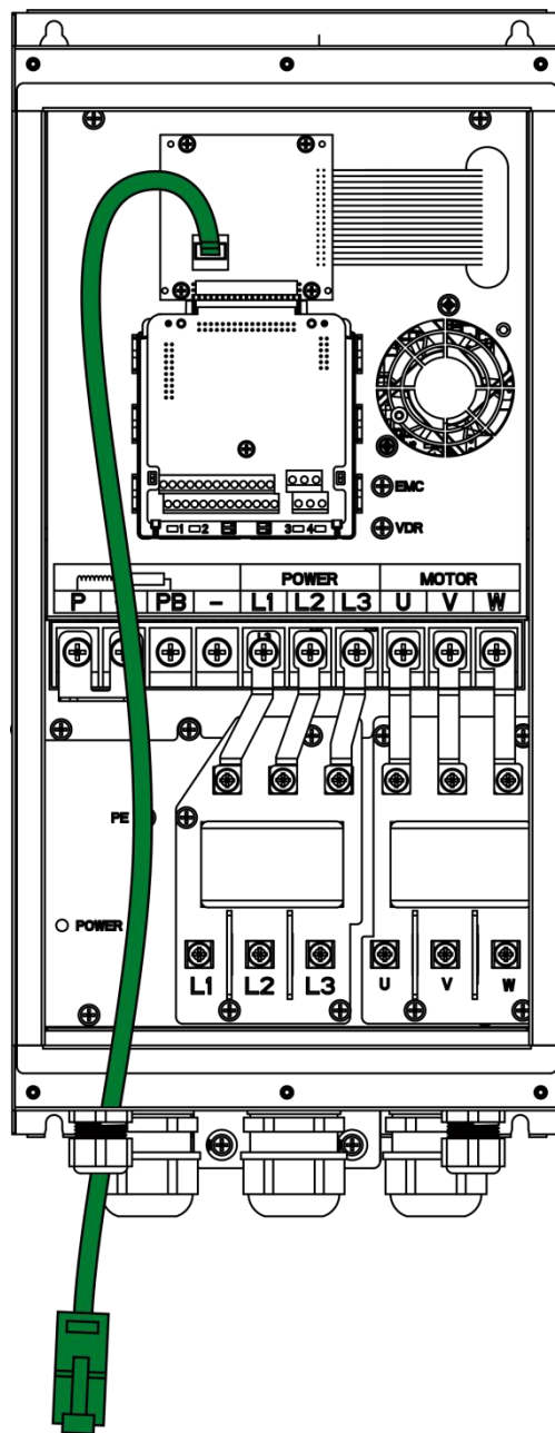
图 3-2 外引键盘网线过线示意图
