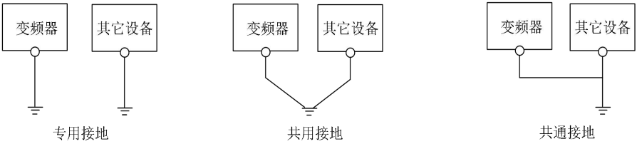
图 3-18 驱动器和其它设备接地方式
