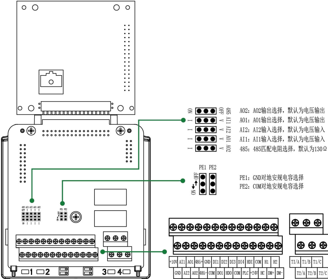
图 3-7 控制回路端子分布图
