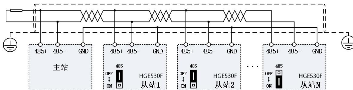
图 3-13 多台变频器 RS485 与上位机连接通信
