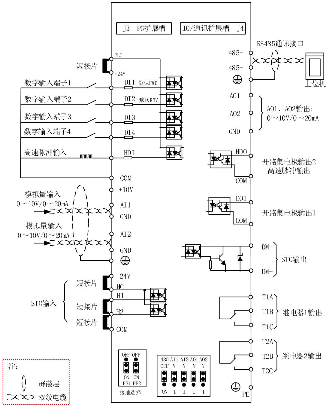
图 3-6 HGE530F 控制回路端子示意图
