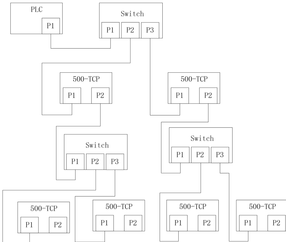
(c) 树形
