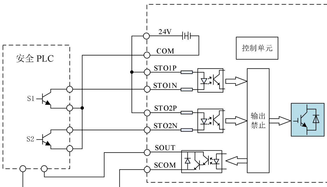
图 3-17 STO 与安全 PLC 接线图(内部 24V、NPN)
