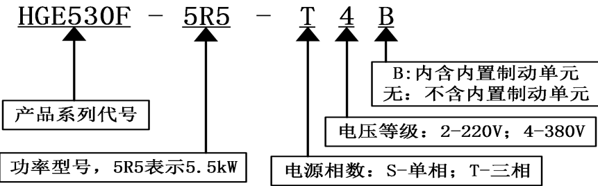
图 2-2 型号说明
