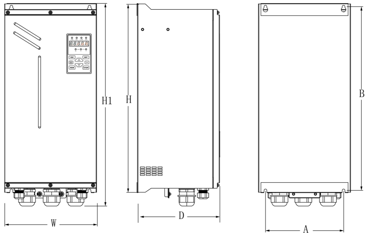
图 3-1 SIZE A～SIZE D（HGE530F-4R0-T4B～HGE530F-045-T4B）外形尺寸图
