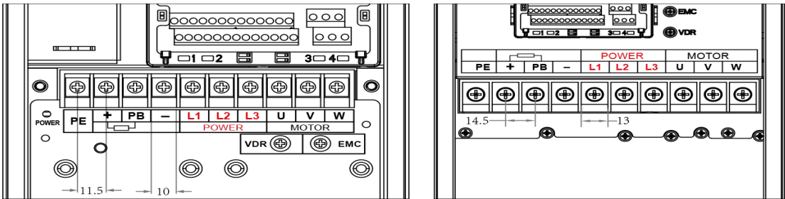
图 3-4 SIZE A~B 主回路接线端子示意图
