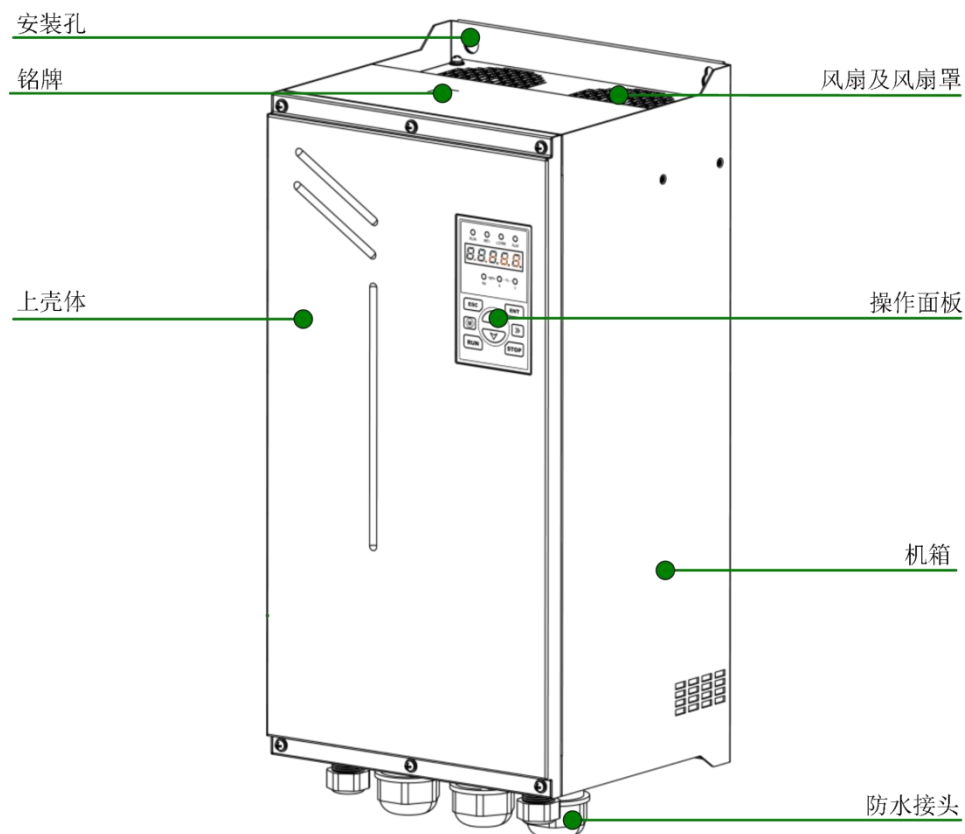
图 2-3 HGE530F 变频器 SIZE A~D (HGE530F-4R0-T4B ~ HGE530F-045-T4B) 部件说明
