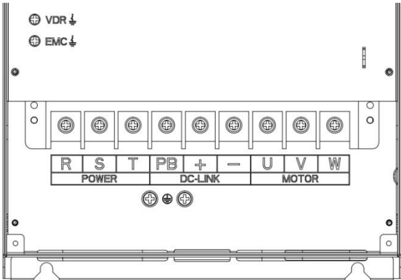
图 3- 12 SIZE F~G 主回路接线端子示意图
