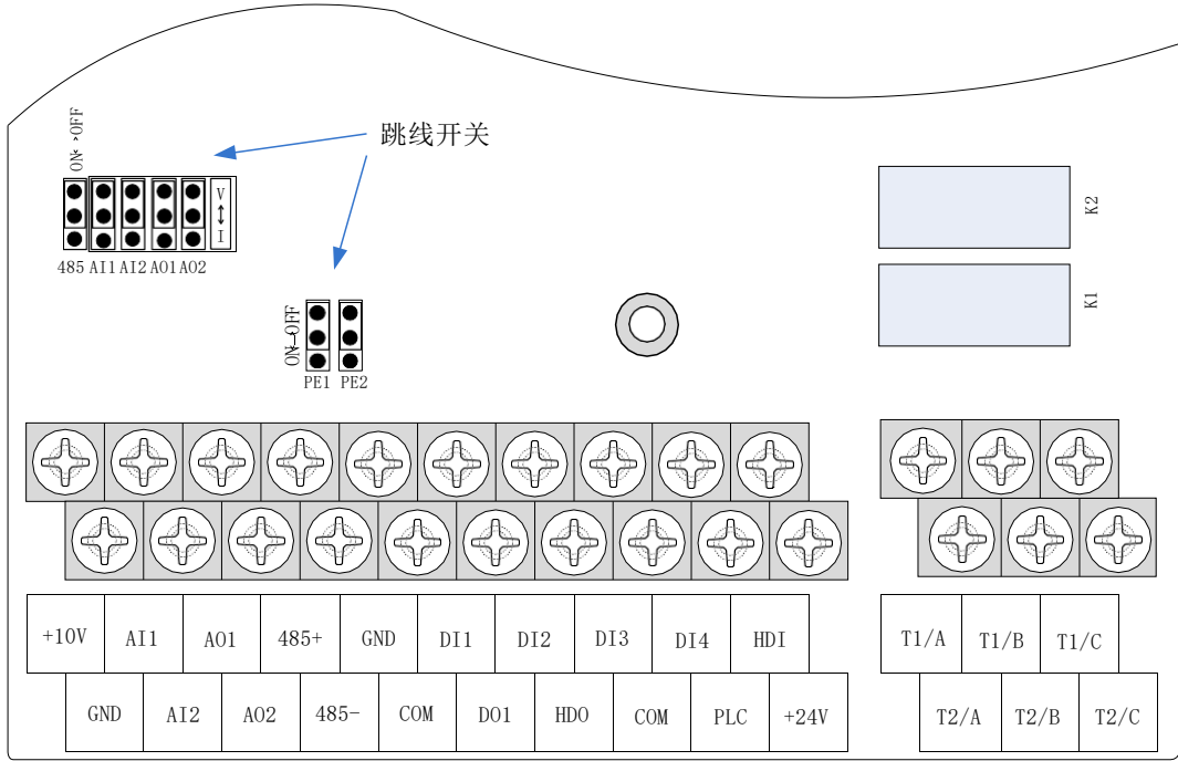
图 3-16 HGE530 控制回路端子示意图
