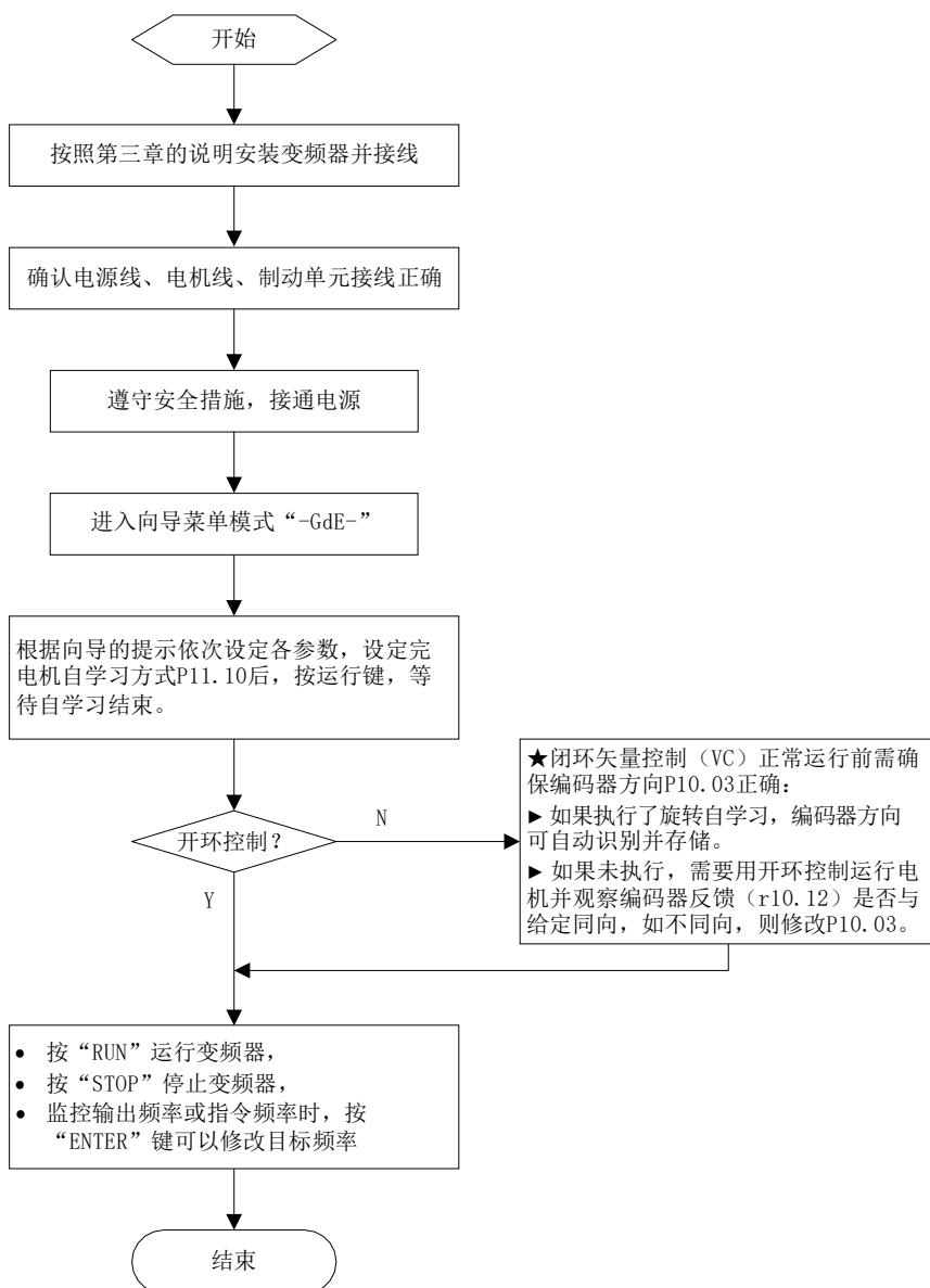
图 4-3 试运行流程图
