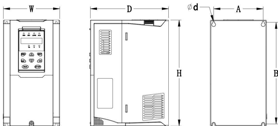
图 3- 4 SIZE A~SIZE C (HGE530-0R7-T4 ~ HGE530-015-T4) 外形尺寸图
