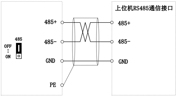
图 3- 21 单台变频器 RS485 直接与上位机连接通信（不接终端电阻）
