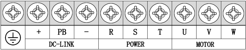
图 3- 9SIZE A~C 主回路接线端子示意图
