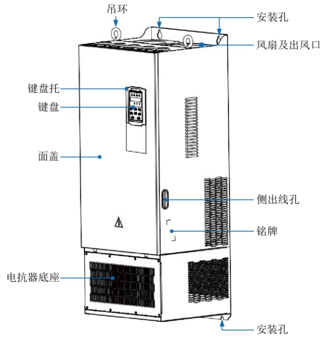
图 2-5 HGE530 变频器 SIZE H ~ SIZE J1 (HGE530-110-T4 ~ HGE530-250-T4) 部件 说明注: SIZE H~SIZE J (HGE530-110-T4 ~ HGE530-200-T4) 机型无电抗器底座
