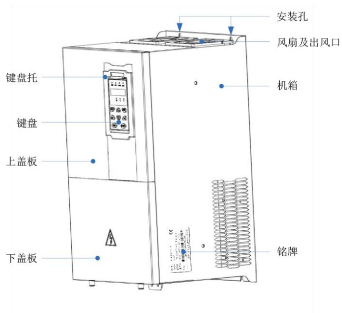
图 2-4 HGE530 变频器 SIZE D~G (HGE530-018-T4 ~ HGE530-090-T4) 部件说明
