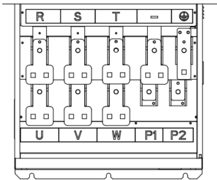
图 3- 14 SIZE K~M（HGE530-280-T4 ~ HGE530-500-T4）主回路接线端子示意图
