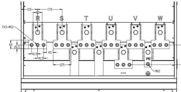
图 3- 15 SIZE N（HGE530-560-T4 ~ HGE530-710-T4）主回路接线端子示意图
