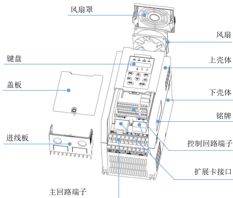
图 2-3 HGE530 变频器 SIZE A~C (HGE530-0R7-T4 ~ HGE530-015-T4) 部件说明
