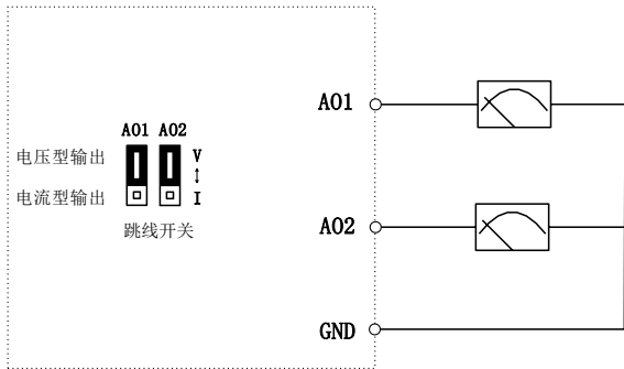
图 3- 18 模拟量输出端子接线图
