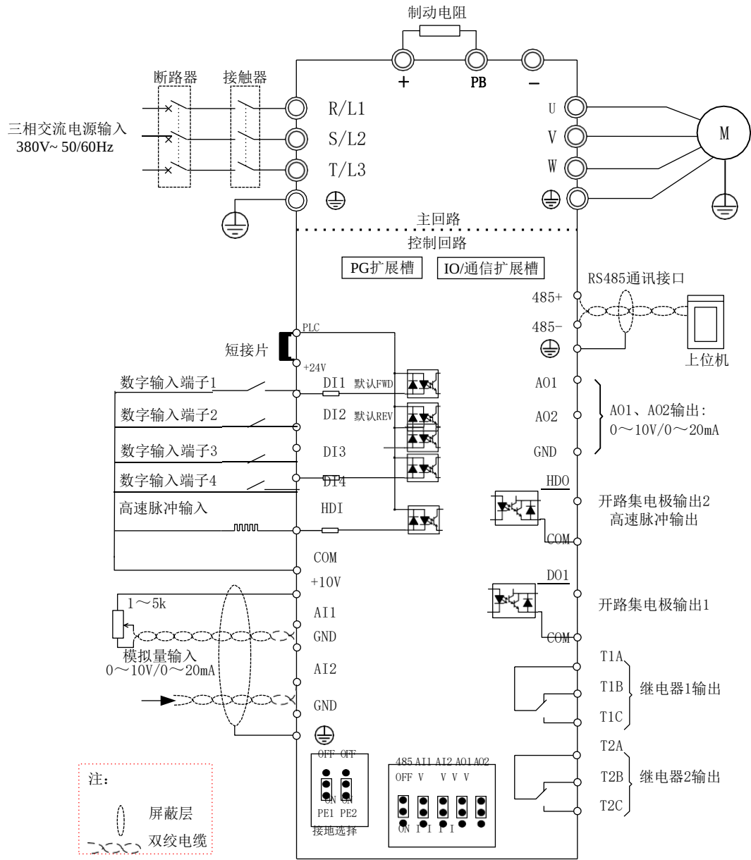
图 3- 8 标准接线图
