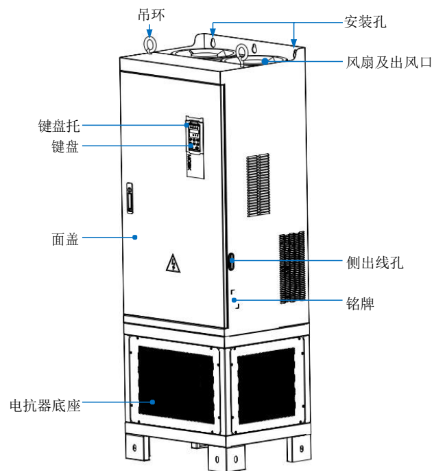
图 2-5 HGE530 变频器 SIZE H ~ SIZE J1 (HGE530-110-T4 ~ HGE530-250-T4) 部件 说明注: SIZE H~SIZE J (HGE530-110-T4 ~ HGE530-200-T4) 机型无电抗器底座
