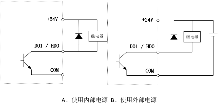
图 3- 20 开关量输出端子接线图
