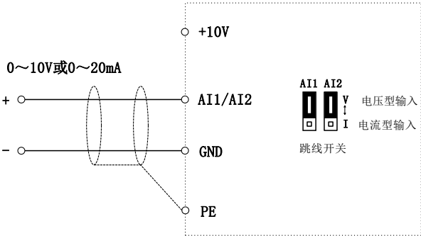
图 3- 17 模拟量输入端子接线图
