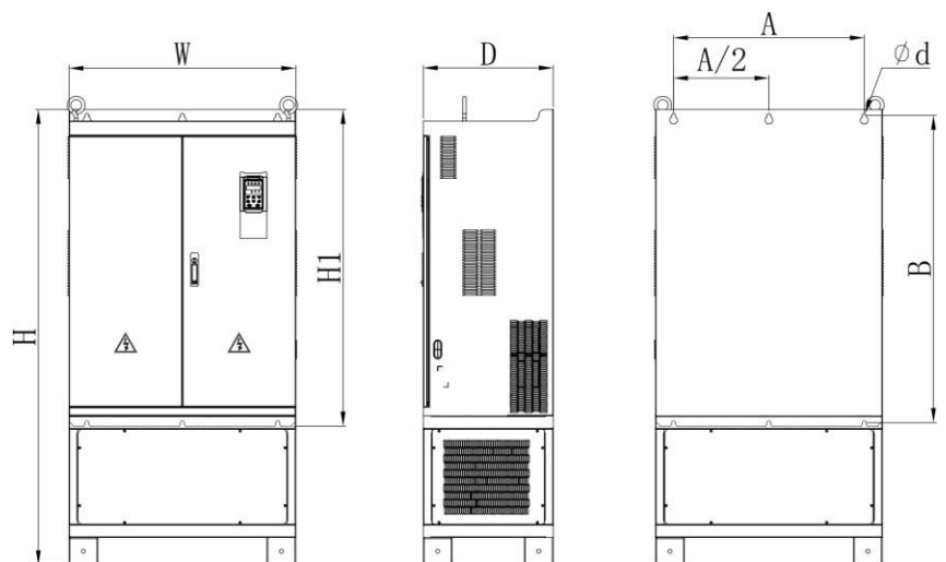
图 3- 8 SIZE L 以上（HGE530-280-T4 以上）外形尺寸图
