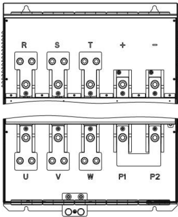
图 3- 13 SIZE H~J1（HGE530-110-T4 ~ HGE530-250-T4）主回路接线端子示意图
