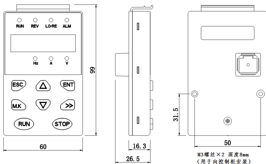
图 3-1 键盘尺寸（单位：mm）
