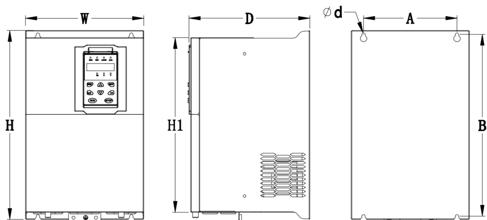
图 3- 5 SIZE D~G (HGE530-018-T4 ~ HGE530-090-T4) 外形尺寸图
