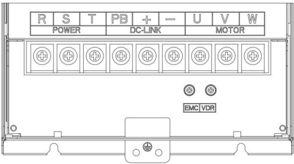
图 3- 11 SIZE E 主回路接线端子示意图
