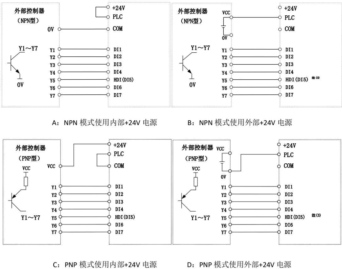
图 3- 19 开关量输入端子接线图
