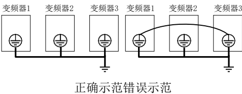
图 3- 23 接地线接法示意图
