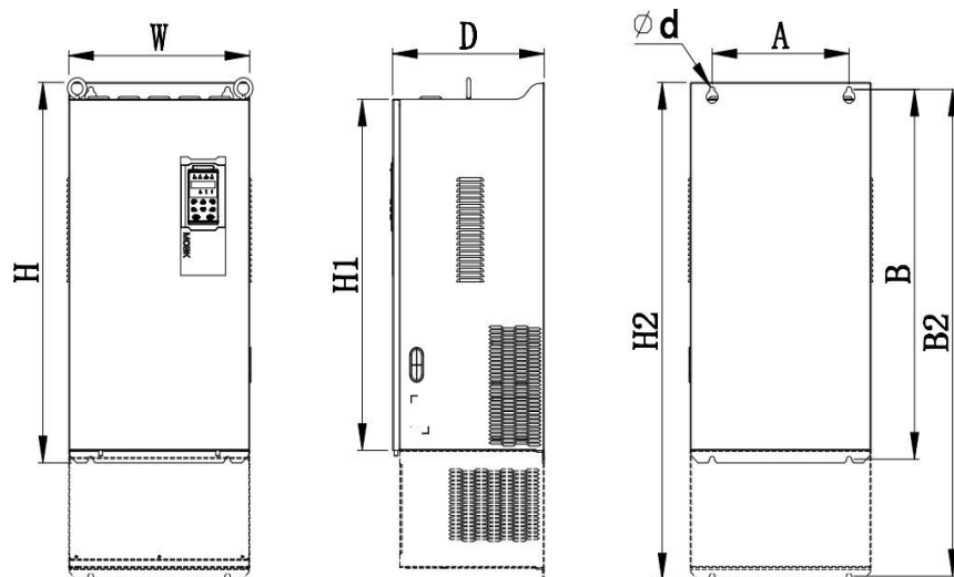
图 3- 6 SIZE H-SIZE J1（HGE530-110-T4 ~ HGE530-250-T4）外形尺寸
