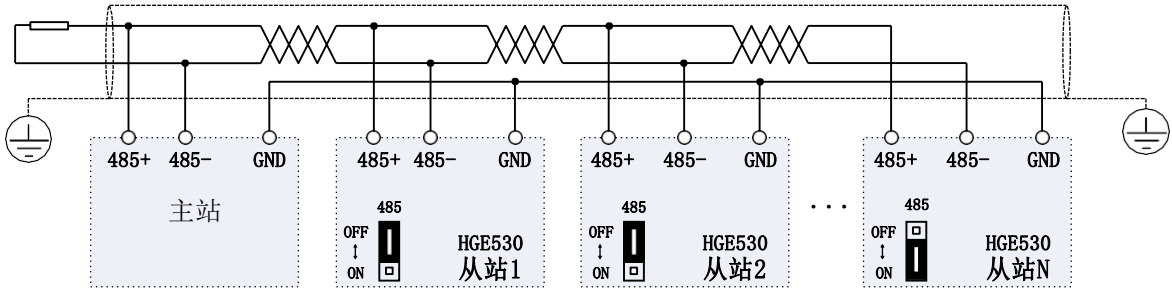
图 3- 22 多台变频器 RS485 与上位机连接通信
