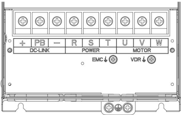
图 3- 10 SIZE D 主回路接线端子示意图
