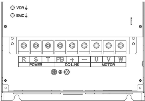
图 3- 16 SIZE F~G 主回路接线端子示意图
