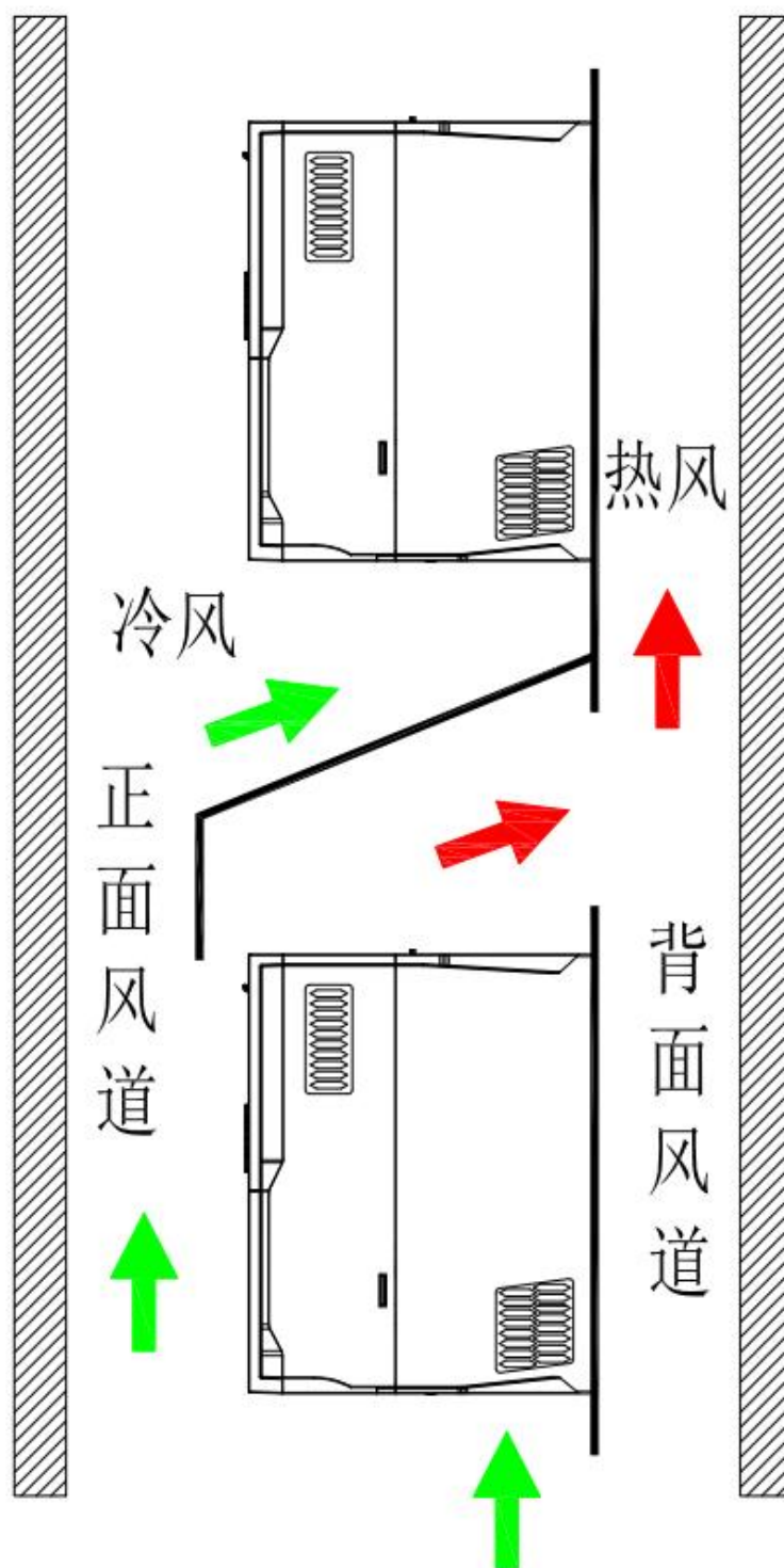
图 3-11 多机上下排安装方向
