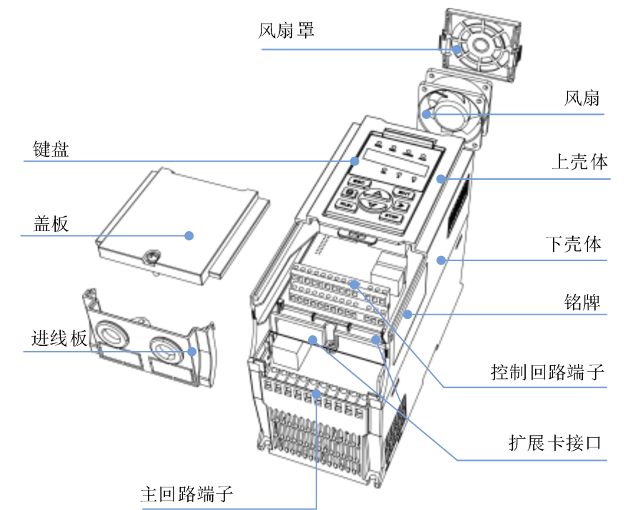
图 2-3 HGE500 变频器 SIZE A~C（HGE500-0R7-T4 ~ HGE500-015-T4）部件说明
