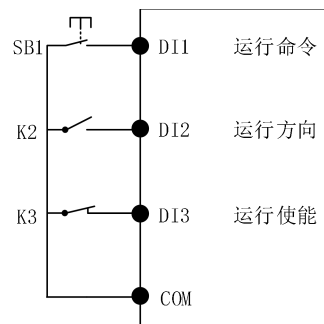
图 4：三线制模式 2
