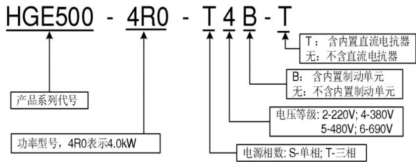
图 2-2 型号说明
