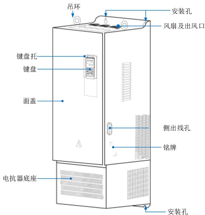
图 2-5 HGE500 变频器 SIZE H ~ SIZE J1 (HGE500-110-T4 ~ HGE500-250-T4) 部件说明
