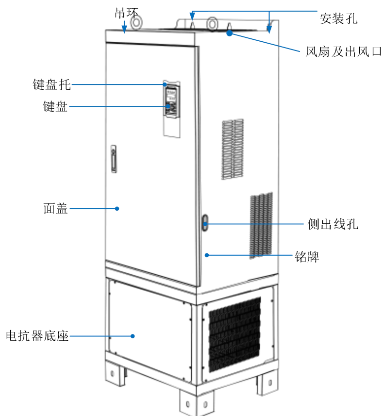
图 2-6 HGE500 变频器 SIZE K ~ N (HGE500-280-T4 ~ HGE500-710-T4) 部件说明
