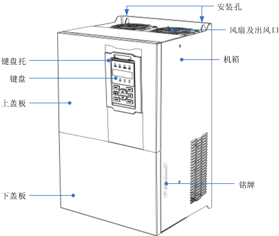
图 2-4 HGE500 变频器 SIZE D~G（HGE500-018-T4 ~ HGE500-090-T4）部件说明
