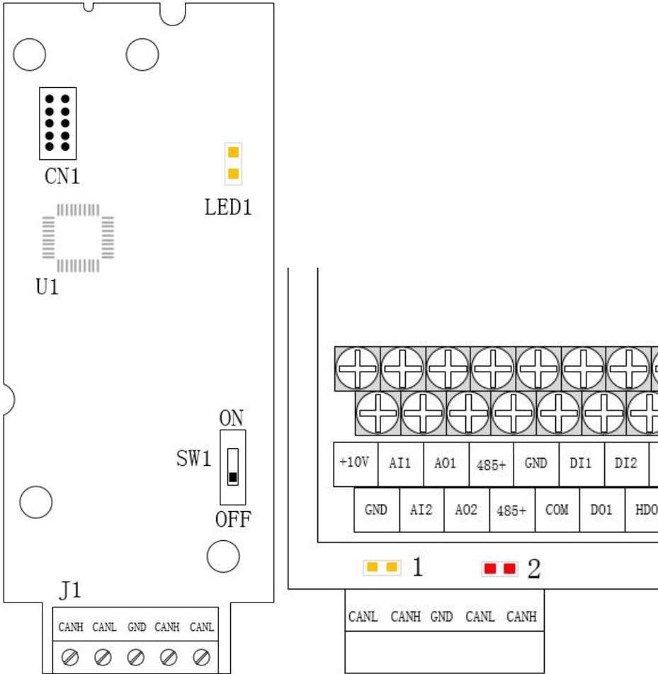
图 7-4 CANopen 通信卡及安装示意图
