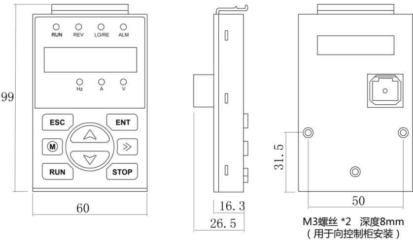
图 3- 1 键盘尺寸（单位：mm）
