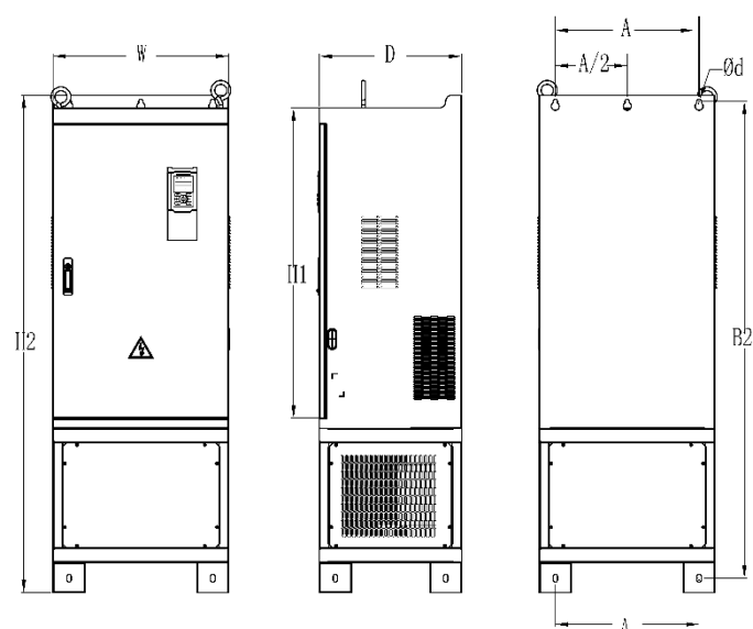
图 3-7 SIZE K (HGE500-280-T4) 外形尺寸图
