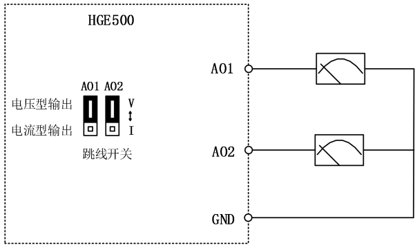
图 3- 22 模拟量输出端子接线图
