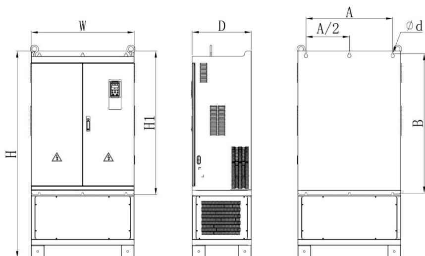
图 3-8 SIZE L 以上 (HGE500-280-T4 以上) 外形尺寸图
