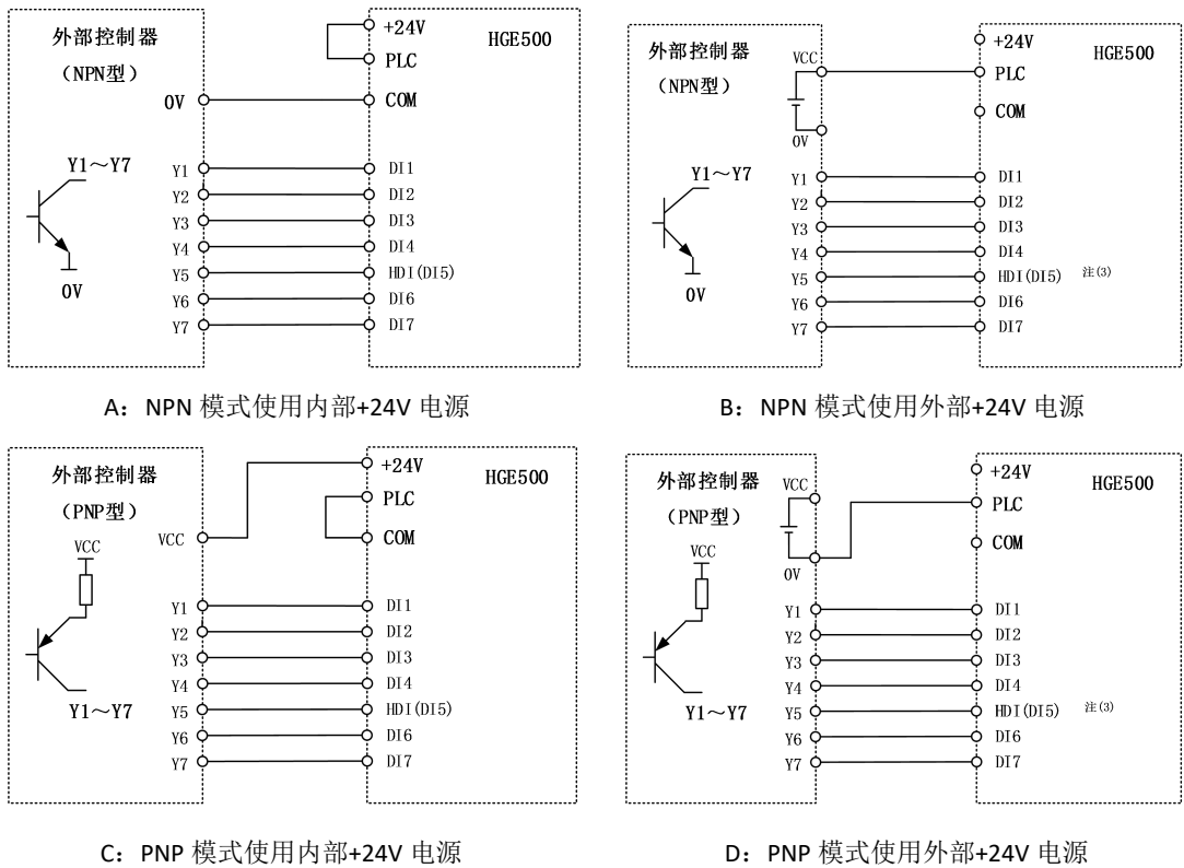
图 3- 23 开关量输入端子接线图
