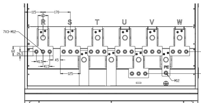
图 3- 19 SIZE N (HGE500-560-T4 ~ HGE500-710-T4) 主回路接线端子示意图
