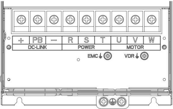
图 3- 14 SIZE D 主回路接线端子示意图
