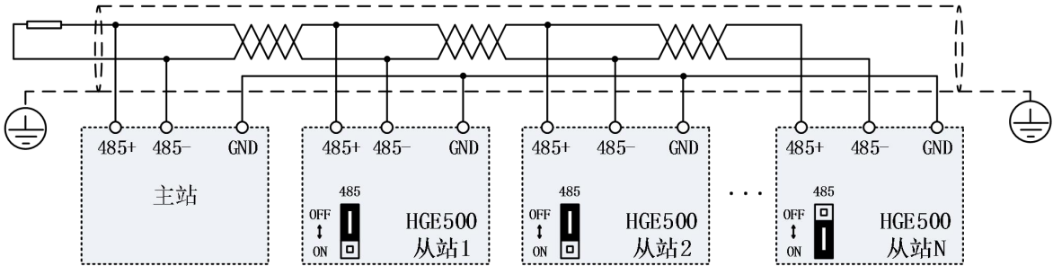
图 3- 26 多台变频器 RS485 与上位机连接通信
