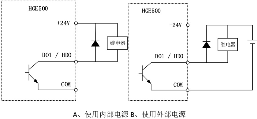
图 3- 24 开关量输出端子接线图
