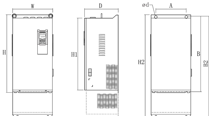
图 3-6 SIZE H~SIZE J1 (HGE500-110-T4 ~ HGE500-250-T4) 外形尺寸图
