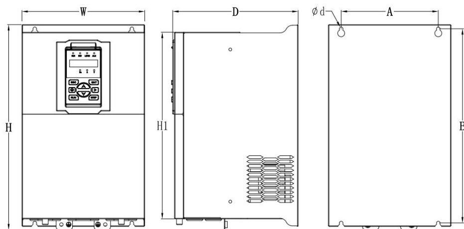
图 3-5 SIZE D~G (HGE500-018-T4 ~ HGE500-090-T4) 外形尺寸图
