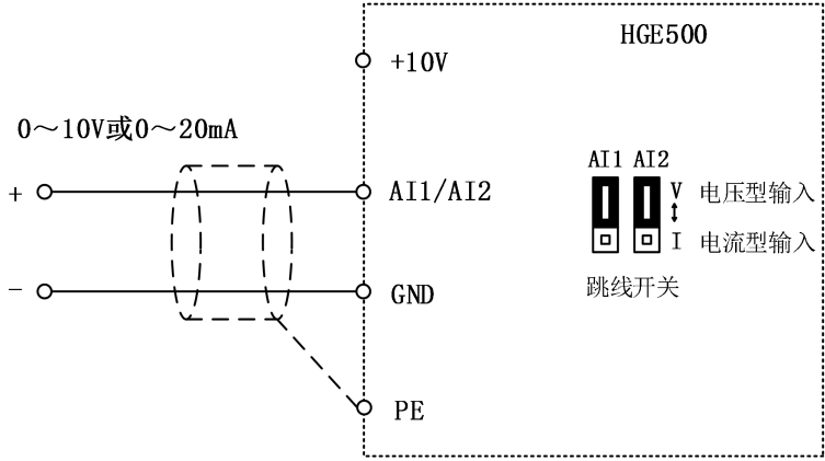
图 3- 21 模拟量输入端子接线图
