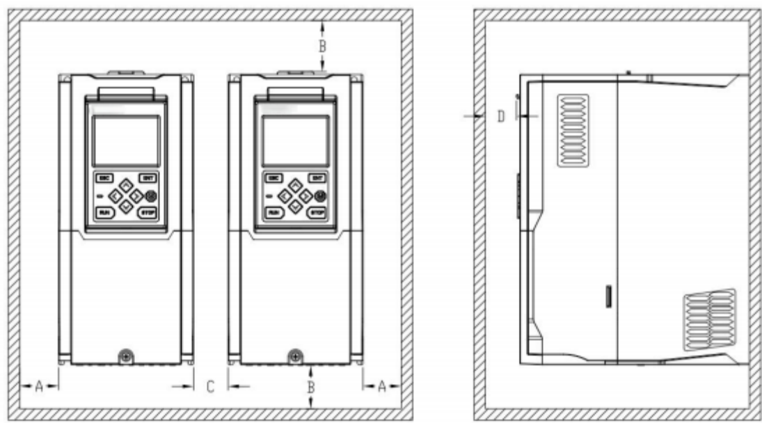
图 3-10 多机并排安装方向和空间（SIZE A～G）
