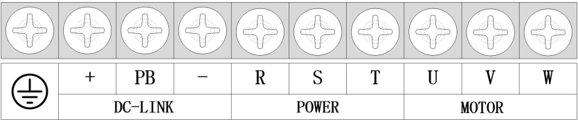
图 3- 13 SIZE A~C 主回路接线端子示意图
