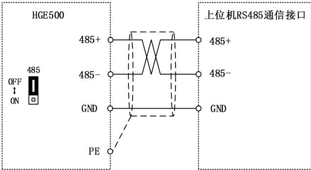
图 3- 25 单台变频器 RS485 直接与上位机连接通信（不接终端电阻）
