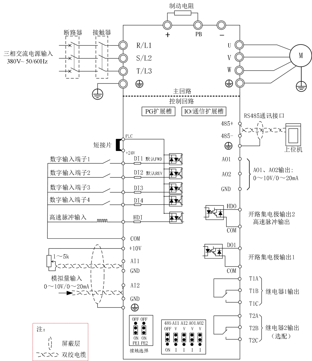
图 3- 12 标准接线图
