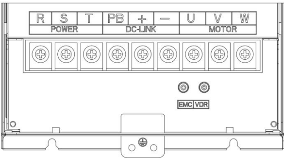
图 3- 15 SIZE E 主回路接线端子示意图
