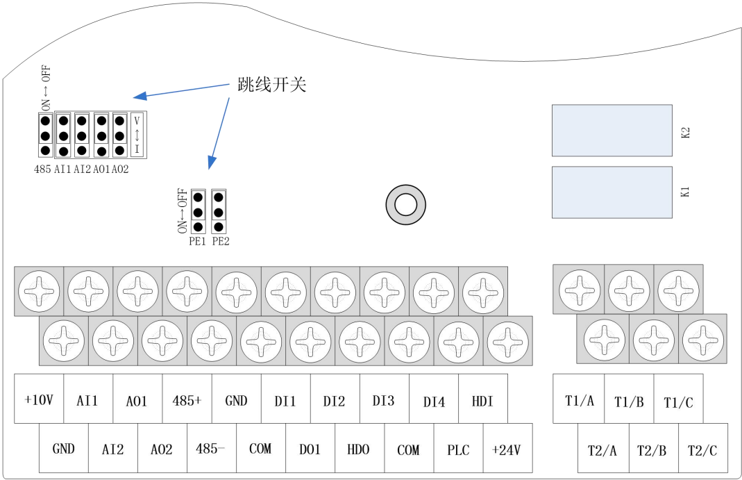
图 3-20 HGE500 控制回路端子示意图
