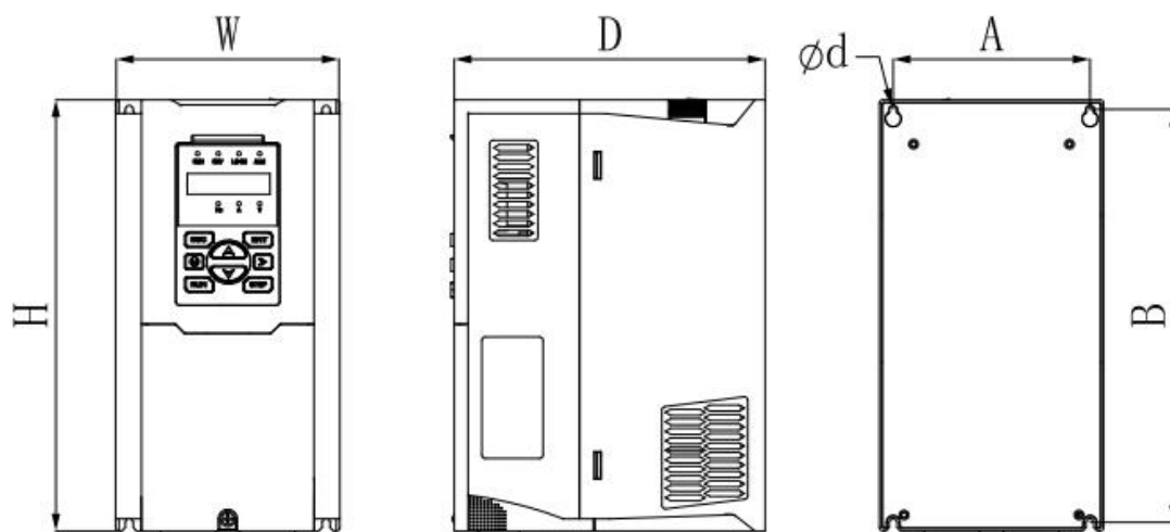
图 3-4 SIZE A~SIZE C (HGE500-0R7-T4 ~ HGE500-015-T4) 外形尺寸图
