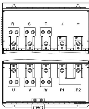
图 3-17 SIZE H~J1 (HGE500-110-T4 ~ HGE500-250-T4) 主回路接线端子示意图
