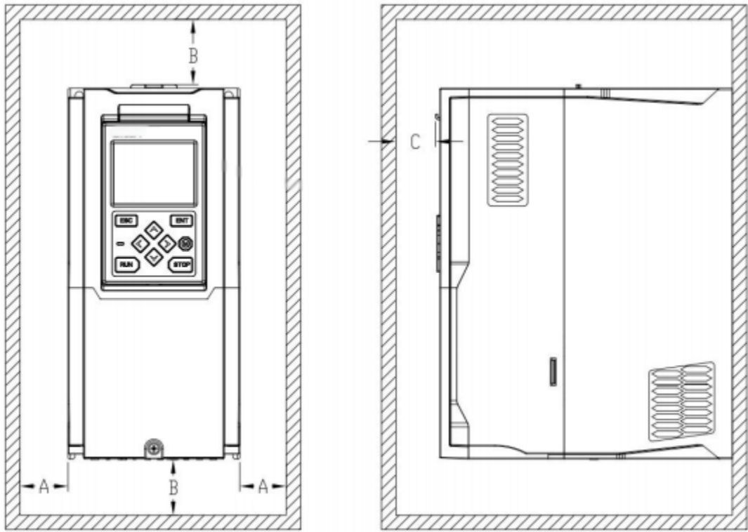
图 3-9 单台驱动器安装空间和方向
