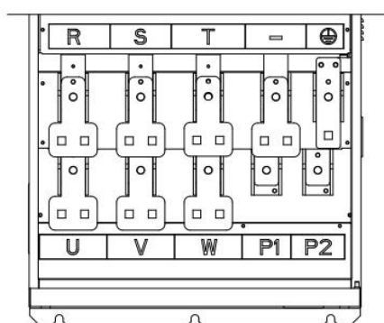
图 3-18 SIZE K~M (HGE500-280-T4 ~ HGE500-500-T4) 主回路接线端子示意图
