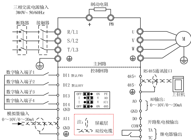
图 3-5 (SIZE A) 标准接线图
