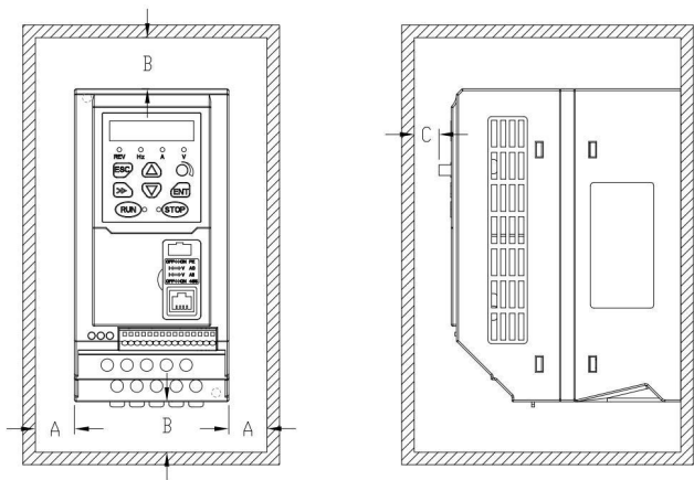
图 3-2 单台驱动器安装空间和方向
