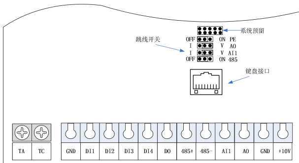
图 3-10 HGE110 控制回路端子示意图 (SIZE A)
