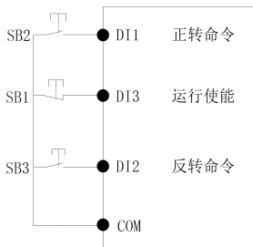
图 3：三线制模式 1
