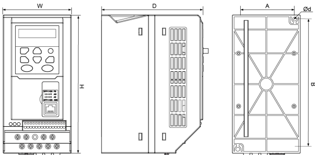
图 3-1 HGE110 SIZE A~C 外形尺寸图
