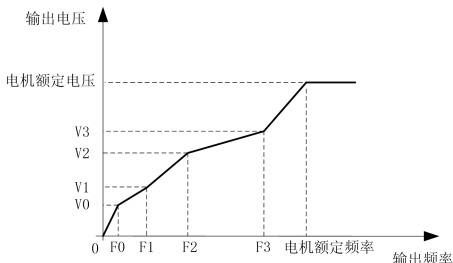
图 2：多段折线型 VF 曲线
