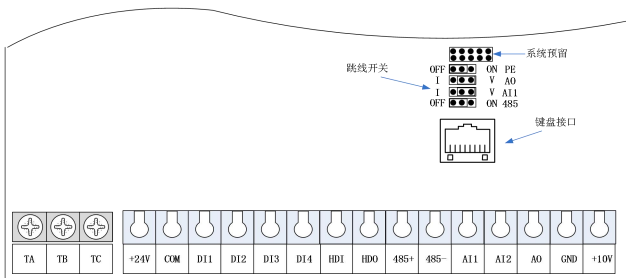
图 3-11 HGE110 控制回路端子示意图 (SIZE B/SIZE C)
