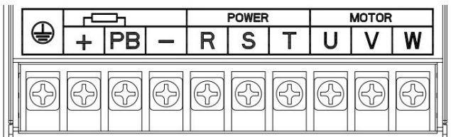
图 3-9 SIZE C 主回路接线端子
