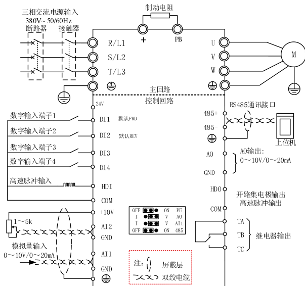
图 3-6 (SIZE B/SIZE C) 标准接线图
