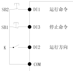
图 4：三线制模式 2
