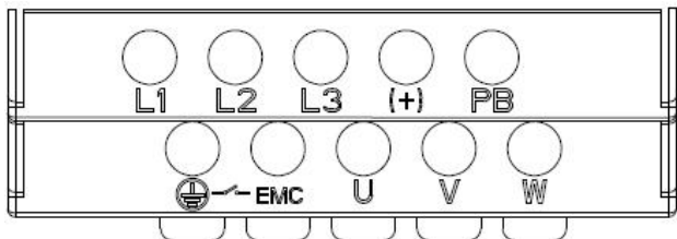
图 3-8 SIZE B 主回路接线端子
