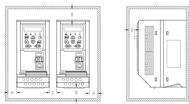
图 3-3 多机并排安装空间和方向
