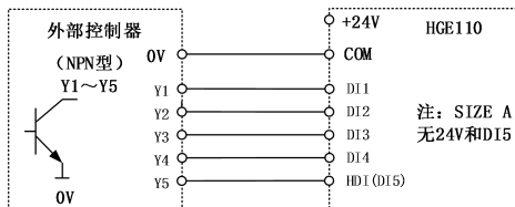
图 3-12 开关量输入端子接线图
