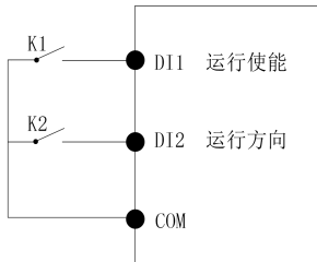
图 2: 二线制模式 2
