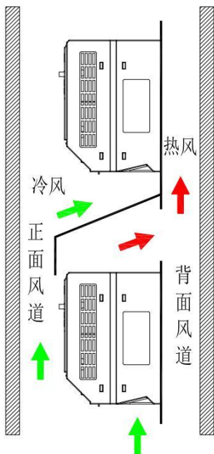
图 3-4 多机并排安装空间和方向
