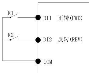
图 1: 二线制模式 1
