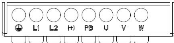
图 3-7 SIZE A 主回路接线端子
