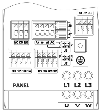
图 3.2 电气接线端子布局
