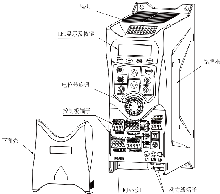
图 2.2 结构示意图（注意个别产品默认无风机）
