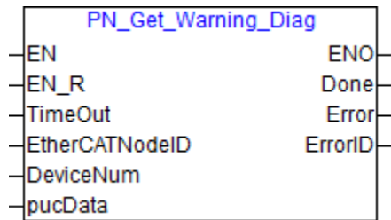
PN_Get_Warning_Diag Functional Block
