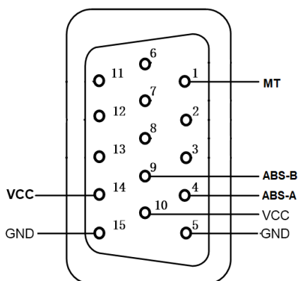
图 2-4 绝对值电机编码器接口定义
