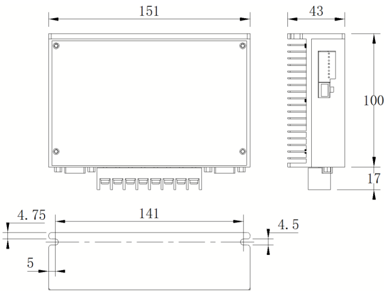
图 1-2 DS/RS20270EA 安装尺寸图 (mm)
