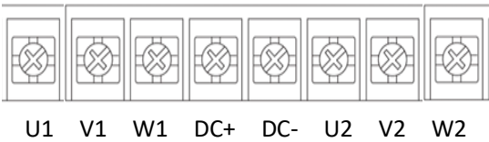
图 2-1 DS/RS20270DA 主回路端子
