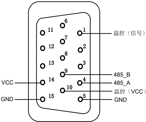
图 2-3 DS20270DA 编码器接口的管脚定义
