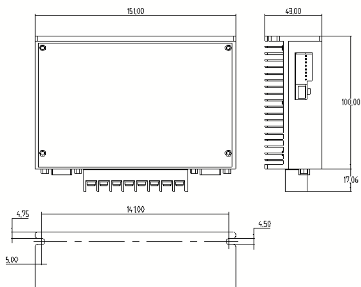
图 1-1 DS/RS20270DA 安装尺寸图
