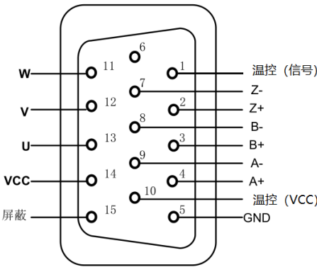
图 2-2 RS20270DA 编码器接口的管脚定义
