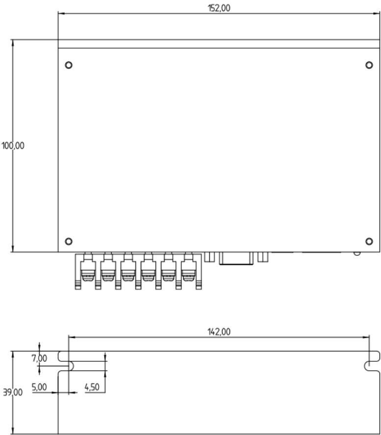
图 1-3 DS/RS10270E 安装尺寸图 (mm)
