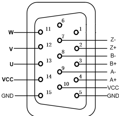
图 2-4 伺服电机编码器接口的管脚定义
