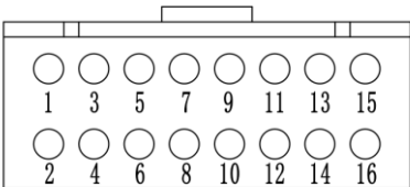
图 2-3 CN3 管脚（母座）
