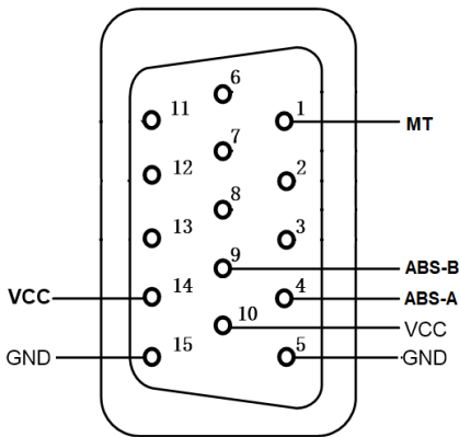
图 2-6 绝对值电机编码器接口定义
