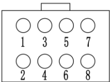
图 2-7 CN6 管脚（母座）
