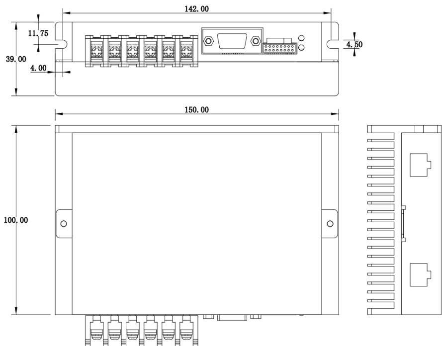
图 1-4 DS/RS10270EB 安装尺寸图（mm）
