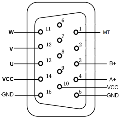
图 2-5 伺服电动轮编码器接口的管脚定义
